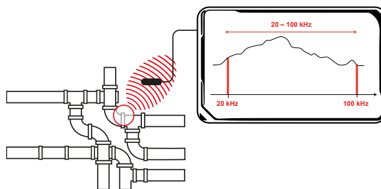
Obr.5: Měření v pásmu 20...100 kHz
